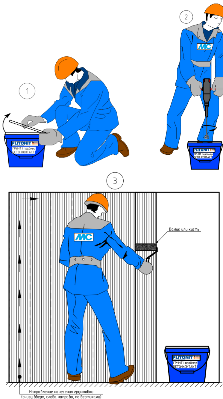
Рис. 11. Последовательность работ.
