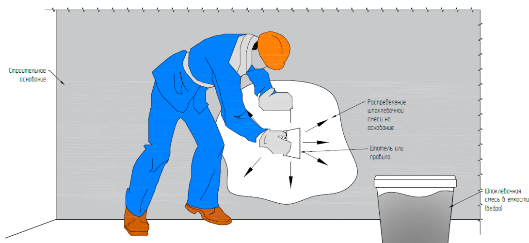
Рис. 23. Организация работ по нанесению шпаклевочной смеси
